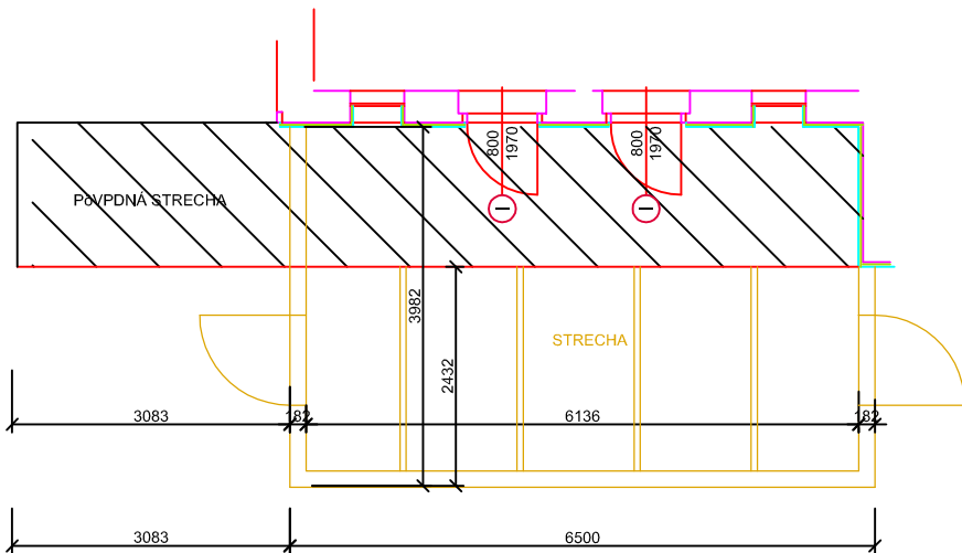
Hliníková strešná konštrukcia s mliečnym polykarbonátom, farba antracit
